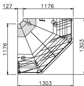
ANGLE 90°: EXTÉRIEUR
