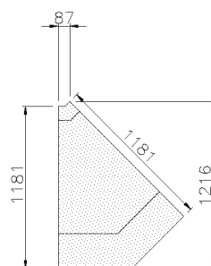
ANGLE 45°: EXTÉRIEUR
