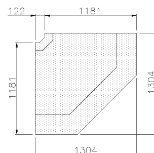
ANGLE 90°: EXTÉRIEUR
