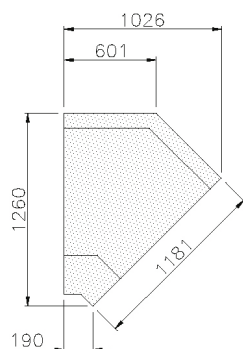
ANGLE 45°: INTÉRIEUR
