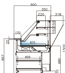
YRSV - VD 3M2 ventilée supérieure
