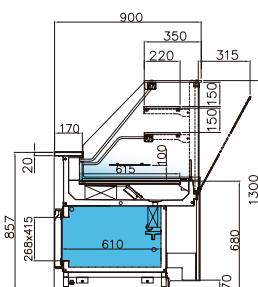
YRTV - VD 3M2 ventilée totale
