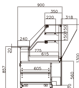
YNO - VD neutre ouverte
