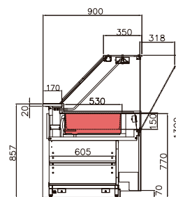
YBM - VD bain-marie
