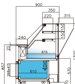
YRTS - VD 3M2 statique totale
