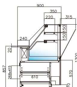
YRSS - VD 3M2 statique supérieure
