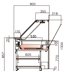
YTAH - VD chaude ventilée avec humidité
