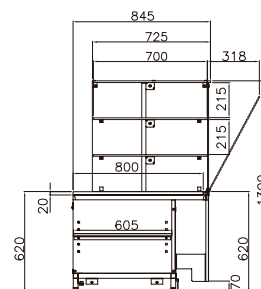
YTV - VD tour vitrée
