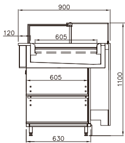
VMINT B - VDB UV neutre
