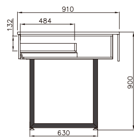
CX1N MIN P caisse
