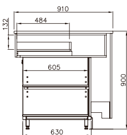
CX1N MIN B caisse
