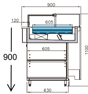
VMINS - VDB UV 3M2 ventilée supérieure
