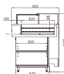
VMINPD B - VDB UV boulangerie
