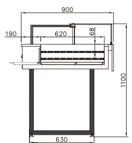
VMINPD P - VDB UV boulangerie
