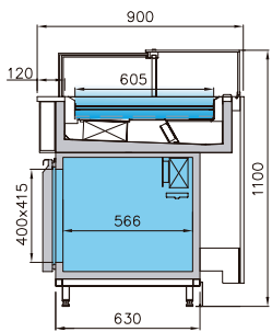
VMINT - VDB UV 3M2 ventilée total
