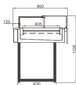
VMINT P - VDB UV neutre
