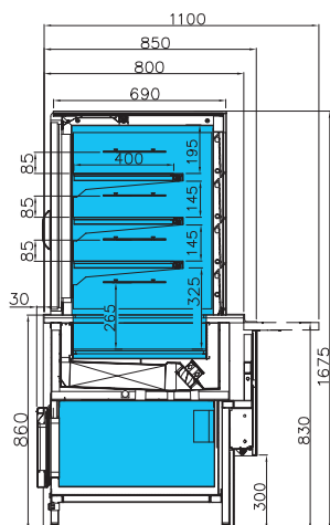
Élément réfrigéré ventilé multi niveaux avec réserve Option rampe à plateaux
