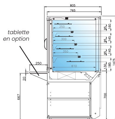
Vitrine réfrigérée réhaussée Vitrage droit
