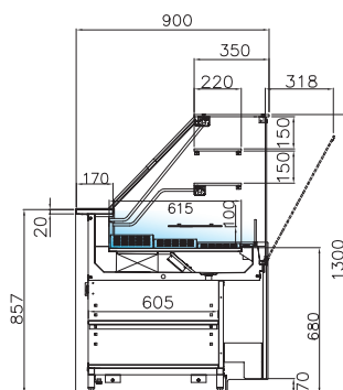
Vitrine réfrigérée Version chocolat / hygrométrie régulée
