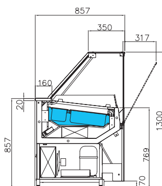
Vitrine réfrigérée Version crème glacée
