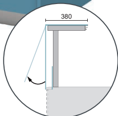
Vitrine plaque chauffante sans réserve + option vitrage relevable
