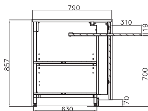
Meuble caisse avec tablette
