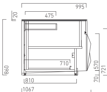
Meuble caisse angle intérieur sans pose-sacs
