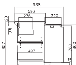
Meuble caisse PMR
