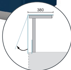
Vitrine neutre + option vitrage relevable
