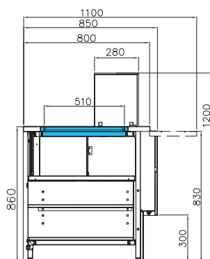
Élément réfrigéré froid contact sans réserve Option vitrage droit et rampe à plateaux
