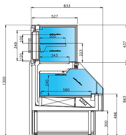
élément réfrigéré ventilé self-service et service arrière
