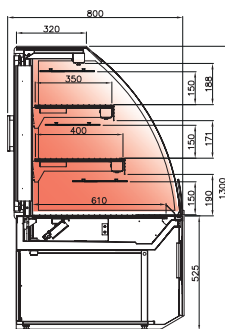
Version chaude ventilée
