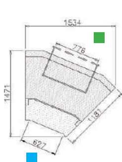
ANGLE 45° : INTÉRIEUR
