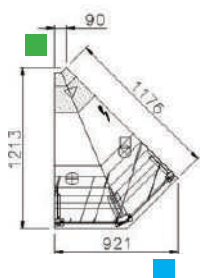
ANGLE 45° : EXTÉRIEUR
