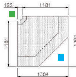
ANGLE 90° : EXTÉRIEUR
