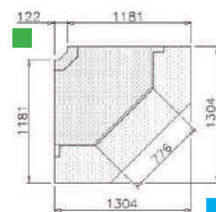
ANGLE 90° : EXTÉRIEUR
