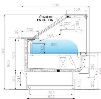
VITRINE RÉFRIGÉRÉE SANS GROUPE
