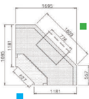
ANGLE 90° : INTÉRIEUR
