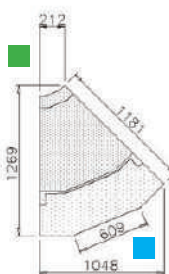
ANGLE 45° : EXTÉRIEUR
